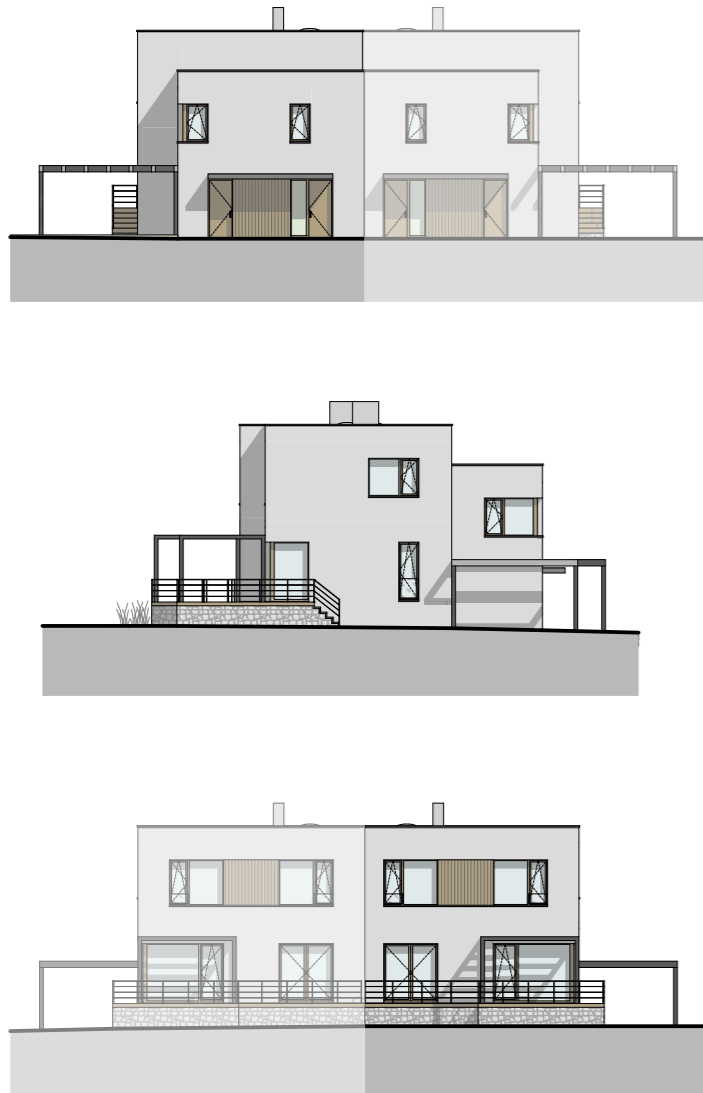
POHLEDY
